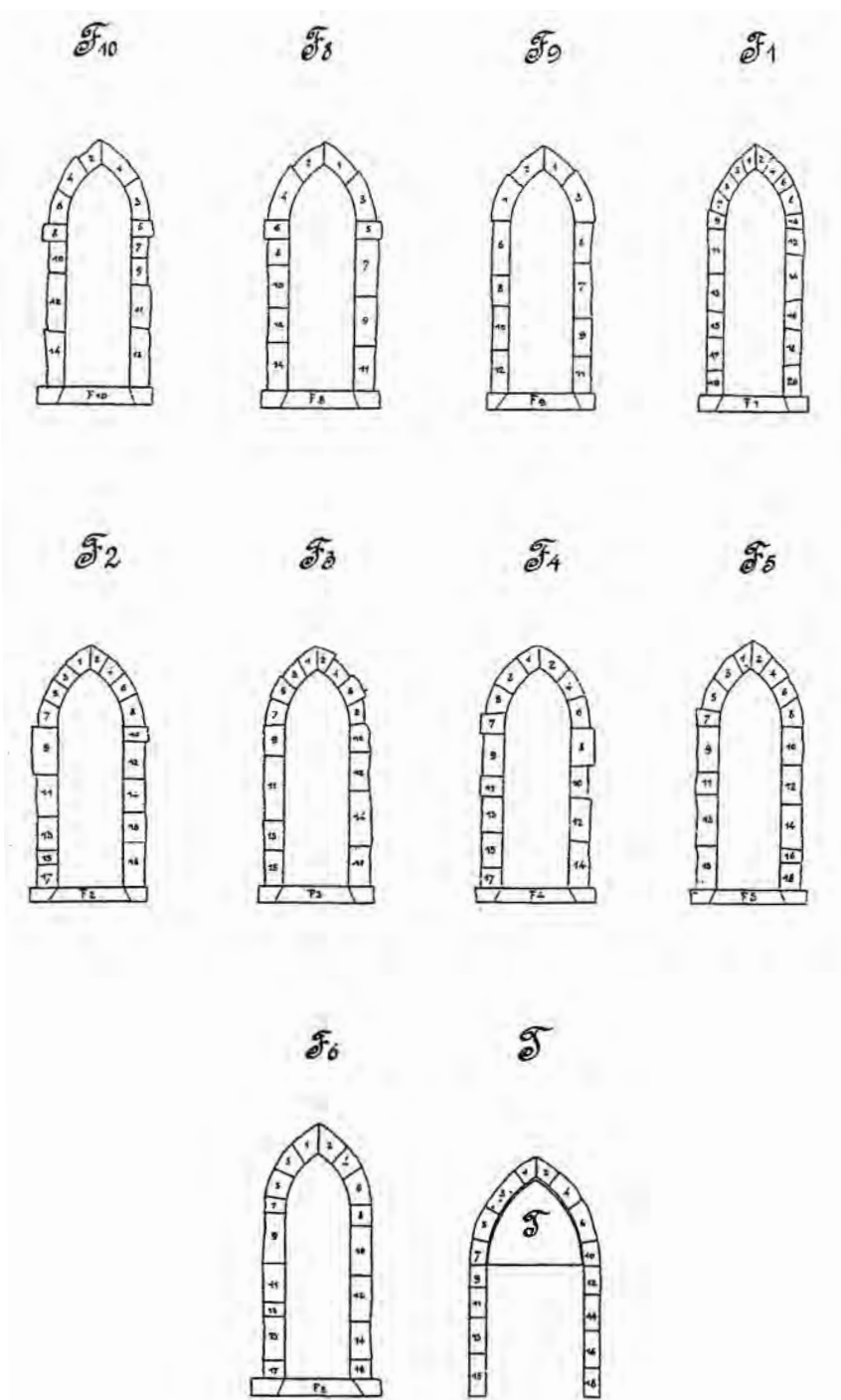
Příloha č. 15: Schématická evidence kamenných bloků oken a vstupního portálu, konec března 1908.
