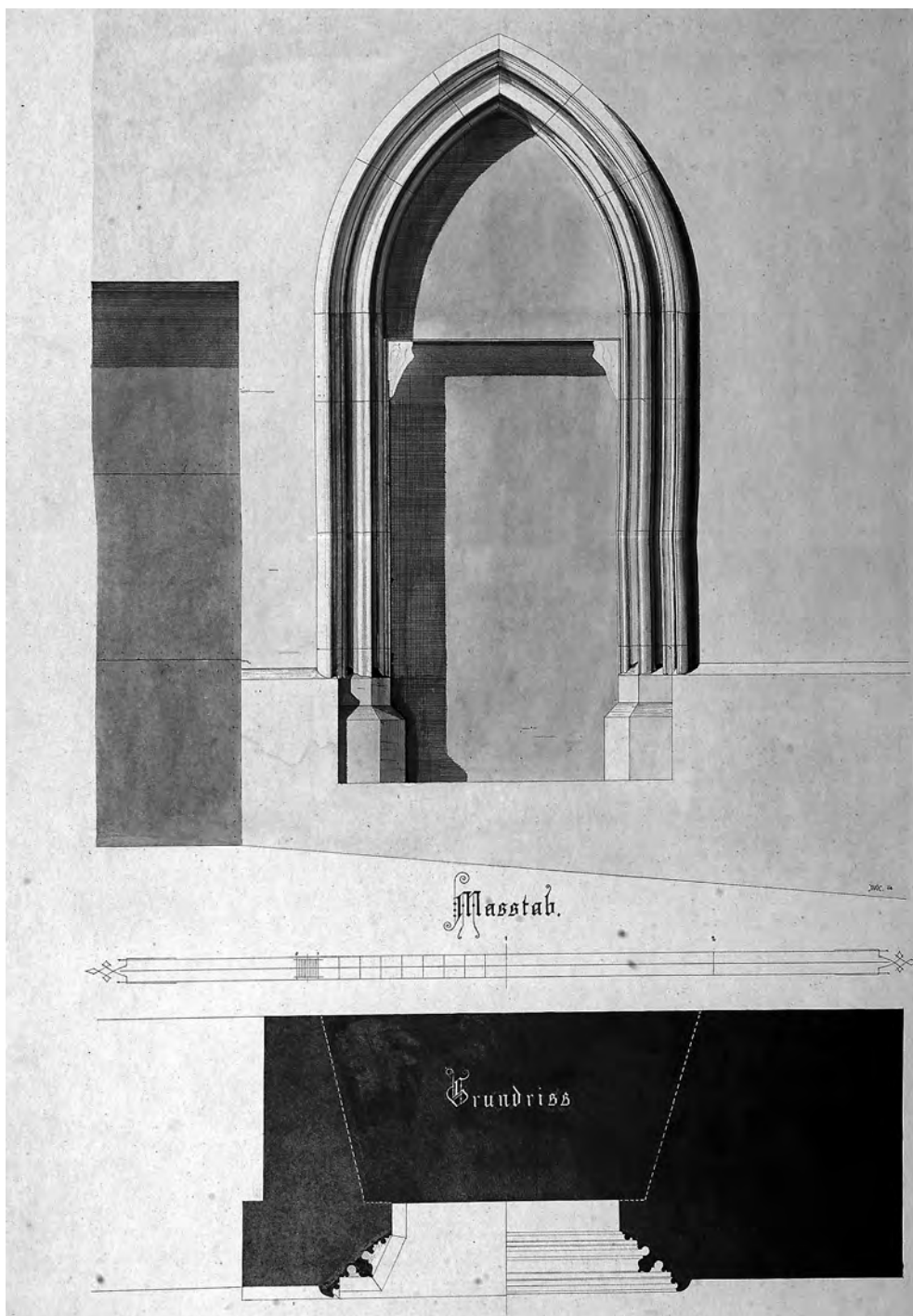
Příloha č. 9: Wilhelm Mayer, Ústupkový portál Královské kaple s plným tympanonem, 1905.
