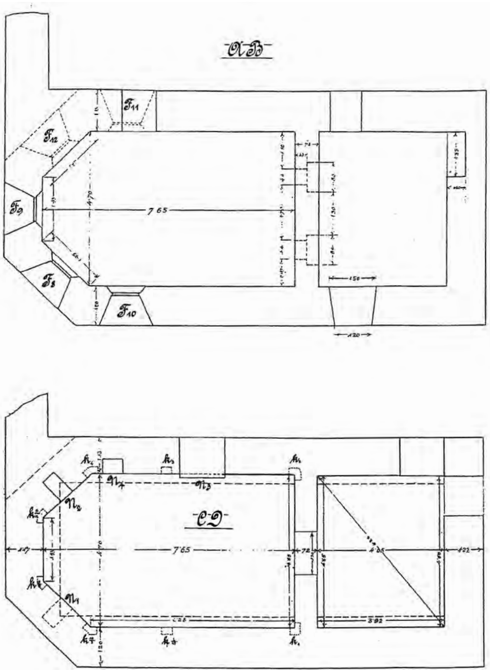
Příloha č. 17: Půdorysy oratoře ve dvou rovinách, A-B ve výšce 500 cm nad podlahou, C-D ve výšce 100 cm nad podlahou, konec března 1908.
